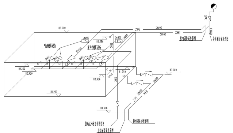
水箱间详图 150
